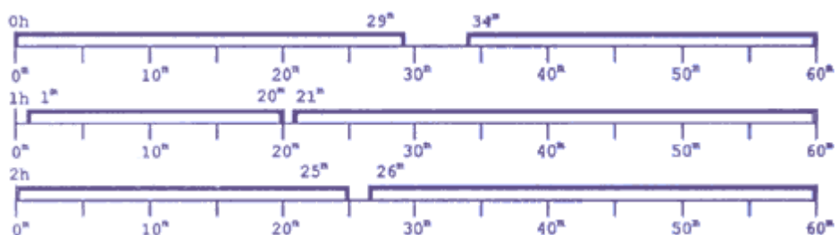
Рис.2. Интервалы звездного времени, в течение которых 4 февраля 1938 г. в Москве не мог родиться человек со Львом на Асценденте
