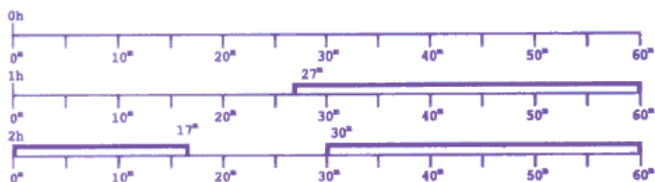
Рис.1. Интервалы звездного времени, в которых вершина I дома не удовлетворяет условиям
