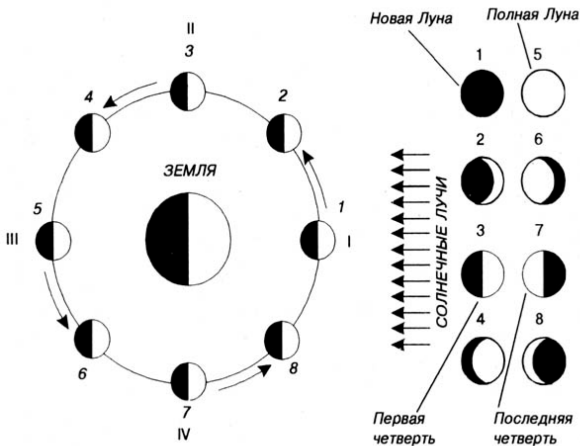
Рис. 3. Фазы Луны
