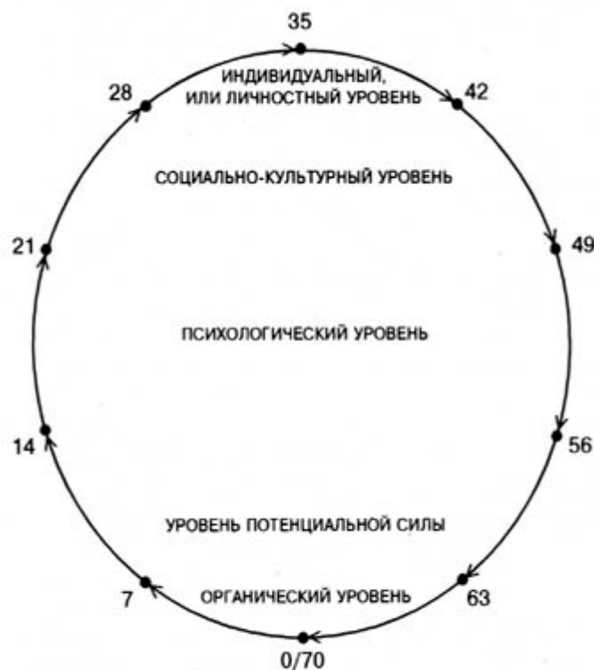
Рис. 2. Цикл семидесятилетней жизни
