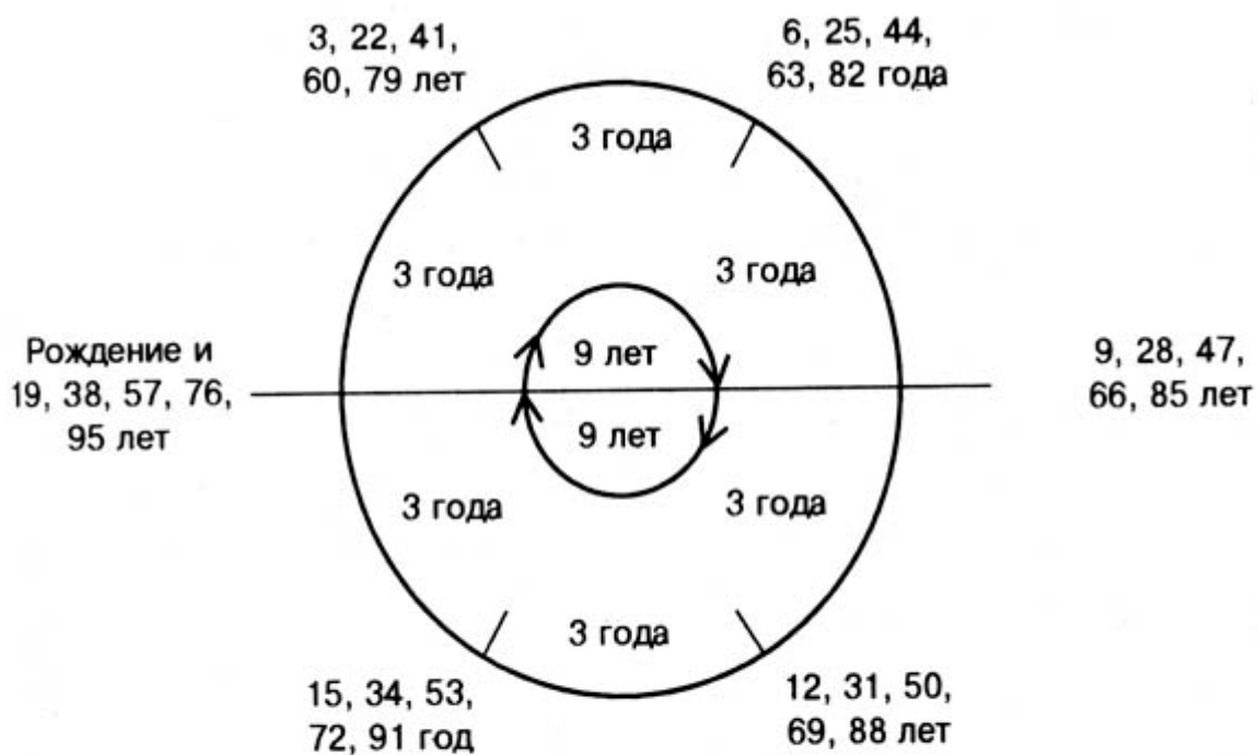
Рис. 5. Деление цикла лунных узлов на трех- и девятилетние периоды
